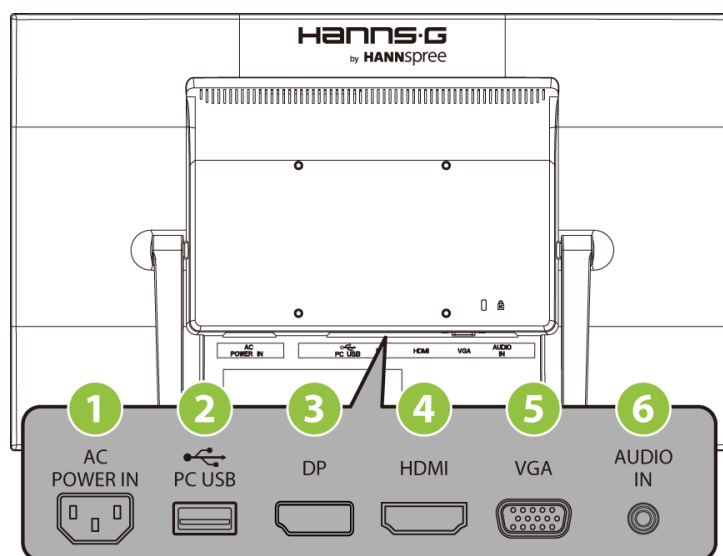
Figura 2. Collegamento al pc
