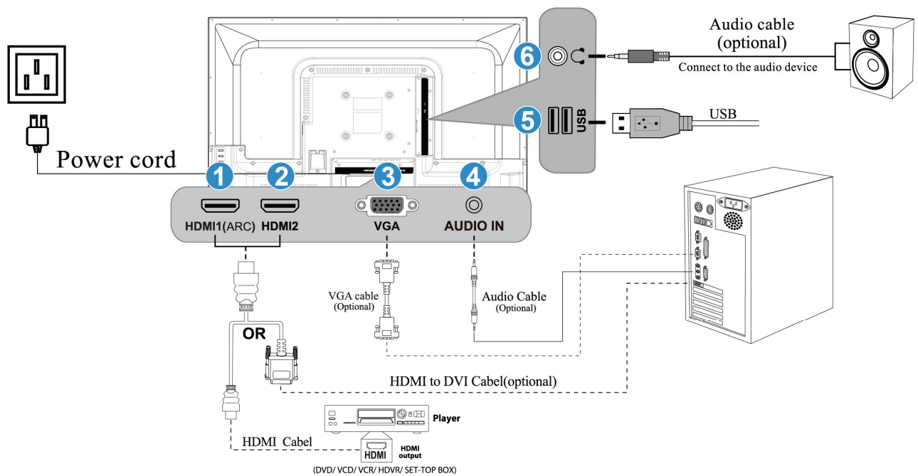
Figura 2. Conexión a un PC
