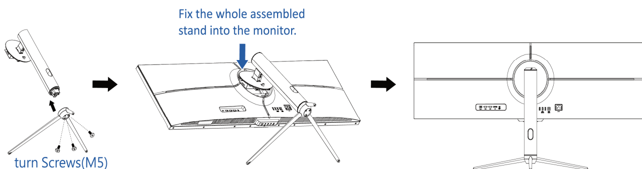
Figure.1. Installer et enlever l'embase
