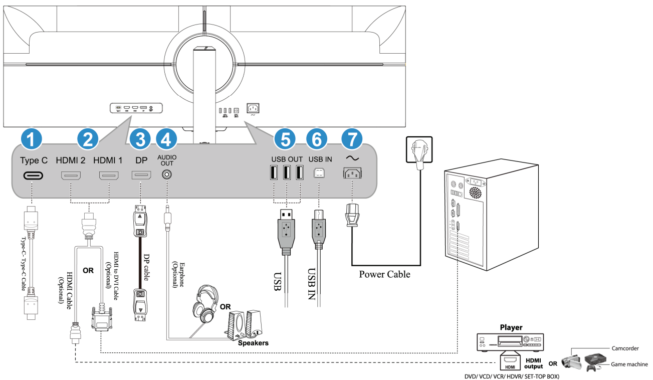
Figura 2. Branchement à un pc
