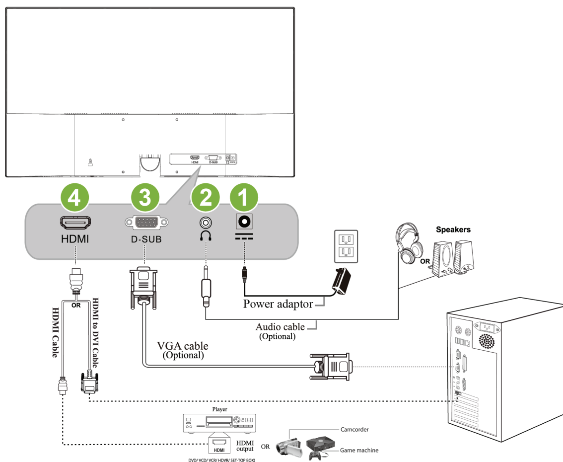
Figura 2. Collegamento al pc
