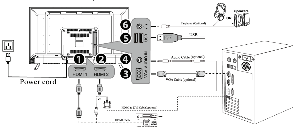
ABBILDUNG 2. ANSCHLISSEN AN EINEN PC
