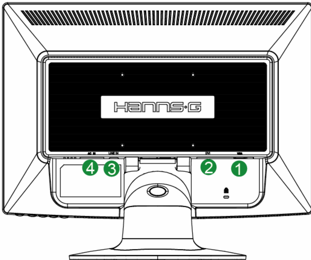
Ilustracja 2 Podłączenia kabli
