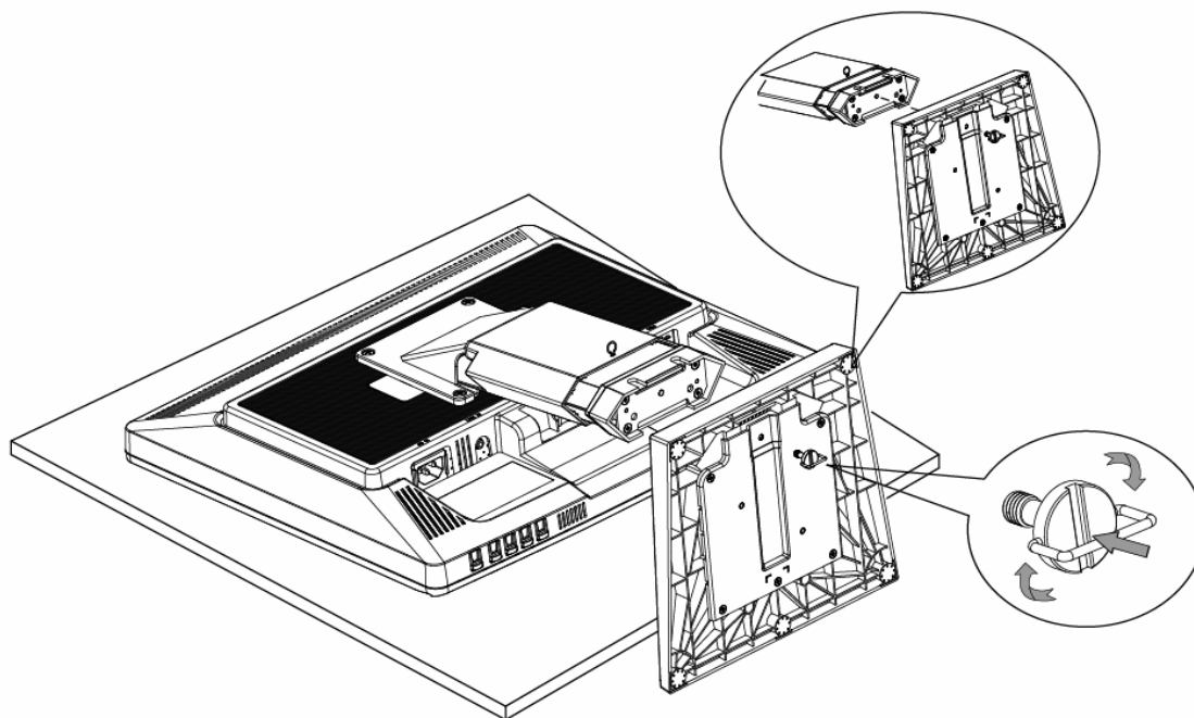
Ilustracja 1 Instalowanie i usuwanie podstawy
