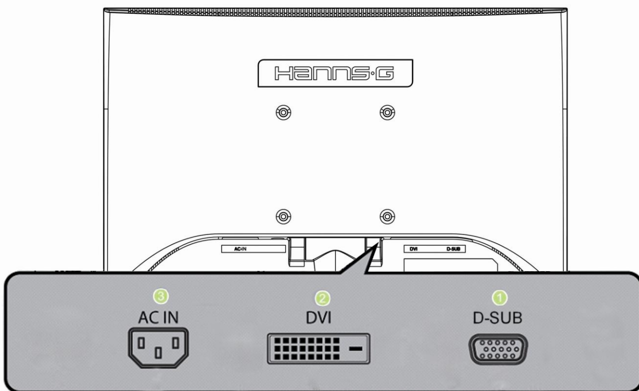
Ilustracja 2 Podłączenia kabli
