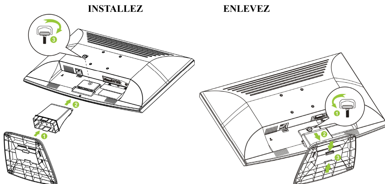
Figure.1. Installer et enlever l'embase
