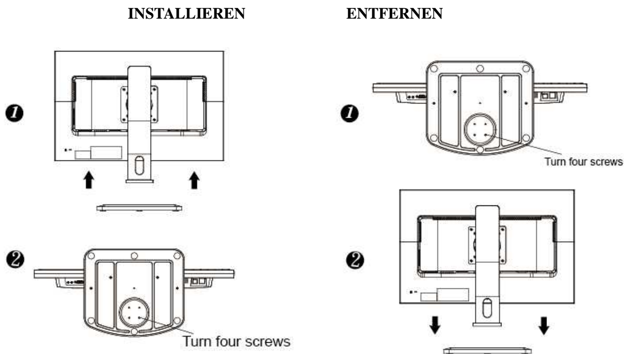
ABBILDUNG 1. INSTALLIEREN UND ENTFERNEN DES STÄNDERS
