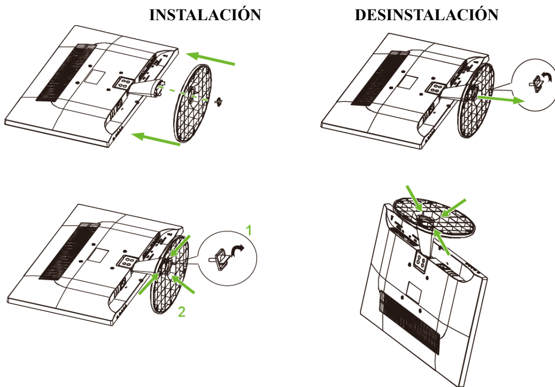
Figura 1. Instalar y desinstalar la base
