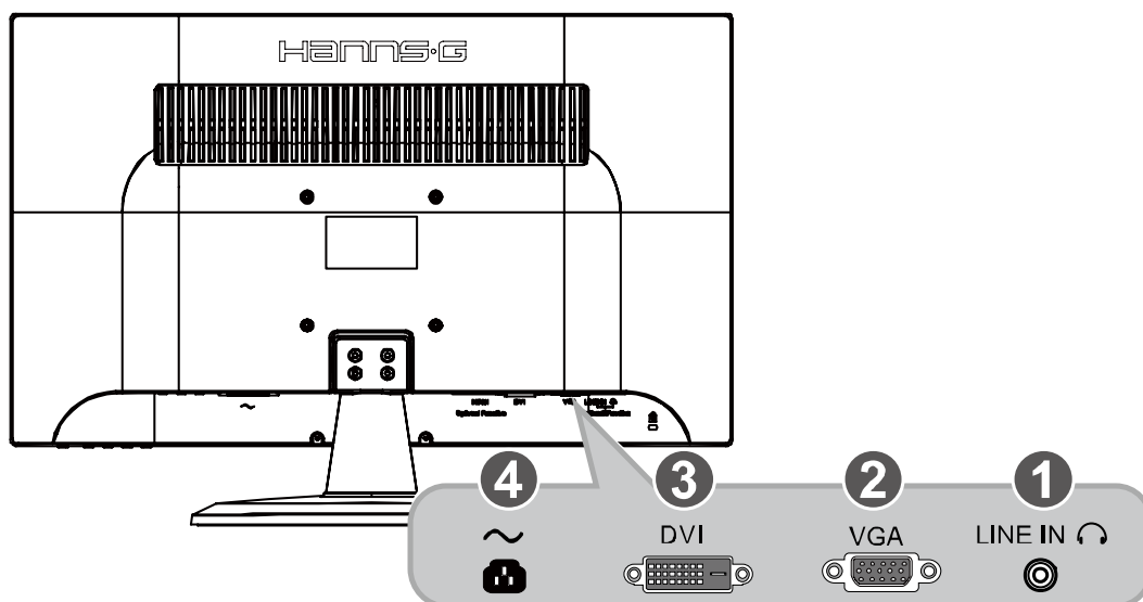
Figura 2. Conexión a un PC
