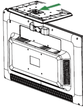
ABBILDUNG 1. INSTALLIEREN UND ENTFERNEN DES STÄNDERS
