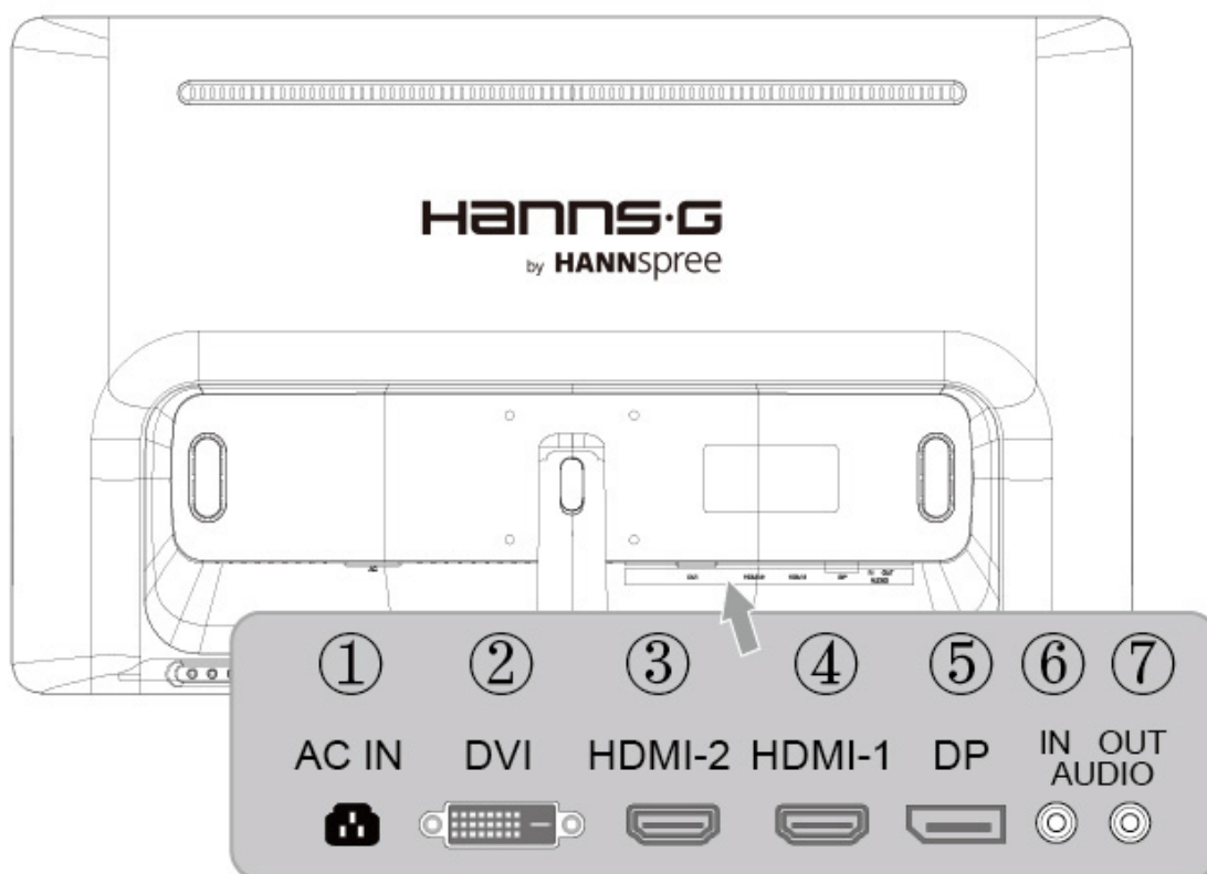
Figura 2. Branchement à un pc
