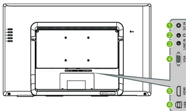
Figura 2. Conexión a un PC
