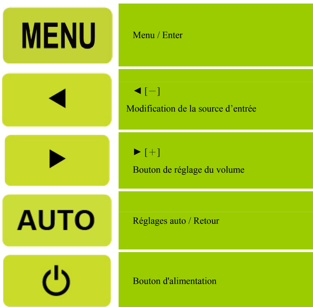
Figure.4. Boutons du panneau de commande
